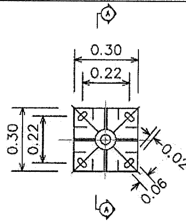
รายละเอียด STEEL BASE PLATE
